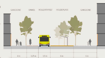
22,75m STRANDVEGEN (SNITT). Det etableres enveiskjørt bussgate sørover i et parti av Strandvegen. Det blir brede fortau, tovegs sykkeltrøpse på gissiden av gaten og stråstille bussoppstillingsplasser for buss på vestsiden. Potensial for fortleng langs gaten.
